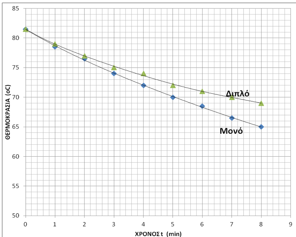
Εικόνα 3. Μεταβολή θερμοκρασίας νερού με τον χρόνο, μονό και διπλό δοχείο
